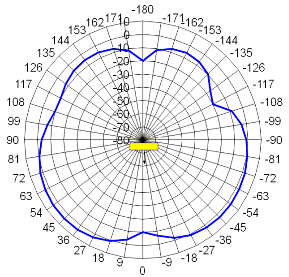
GSM 2100 MHz
