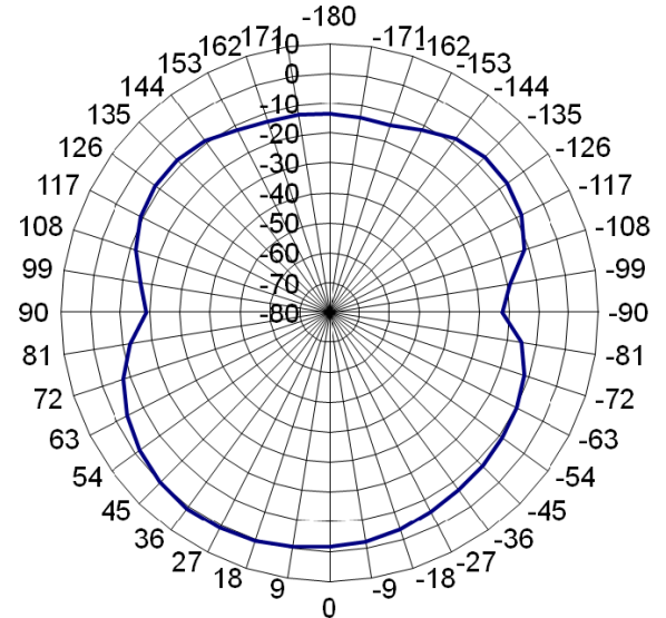
GSM 2100 MHz
