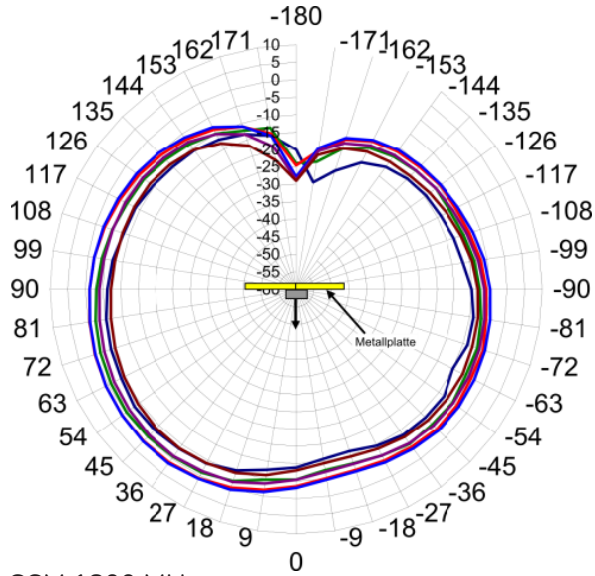
GSM 1800 MHz
